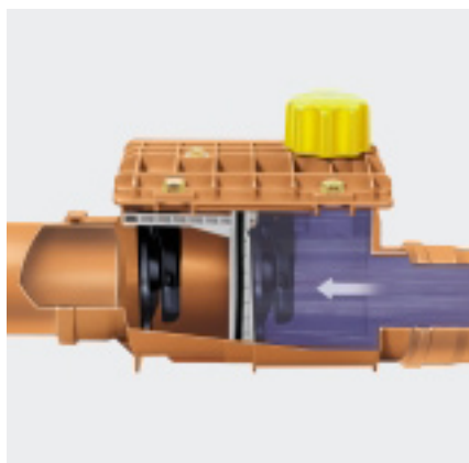
Funkcioniranje nepovratnog ventila – 4986.2
